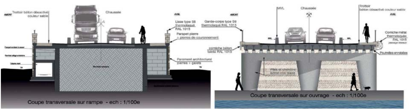
Coupes transversales
