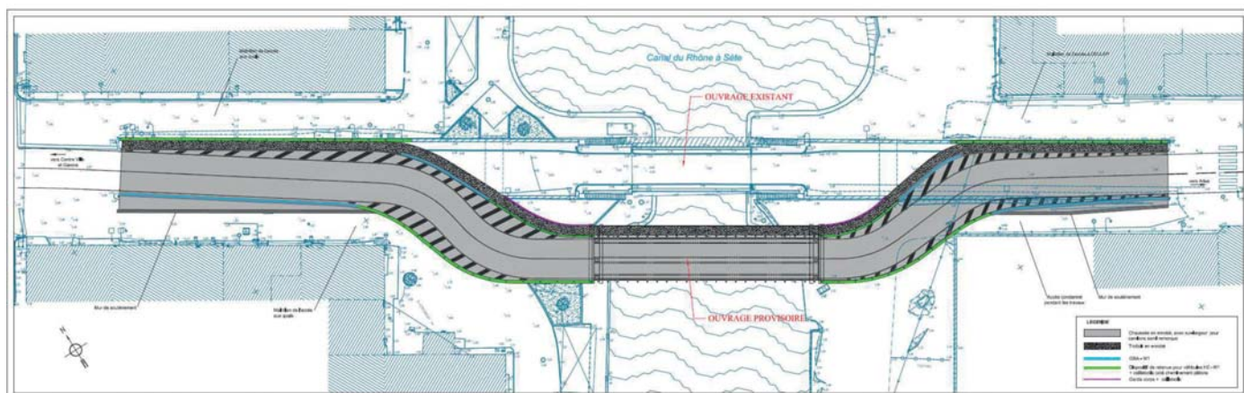
Plan de surface de la déviation provisoire
